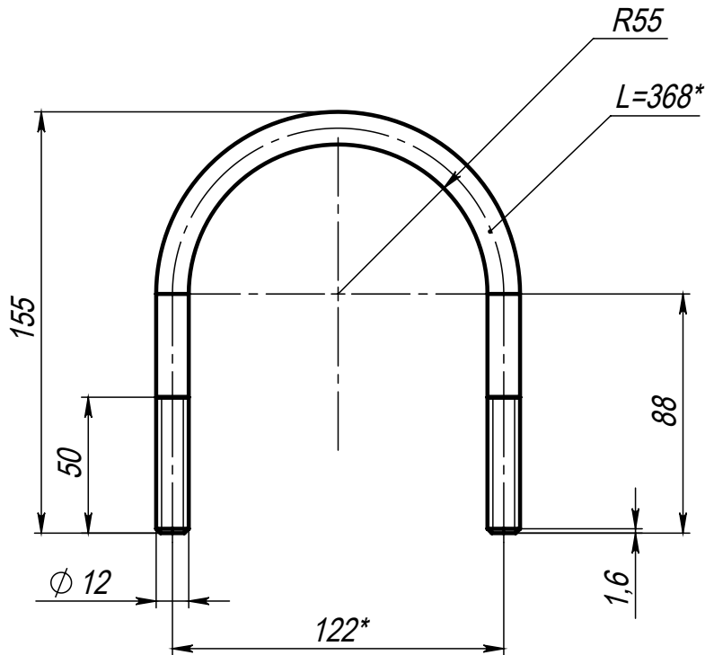
Поз.2 (Хомут)
